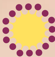
固定化病毒
